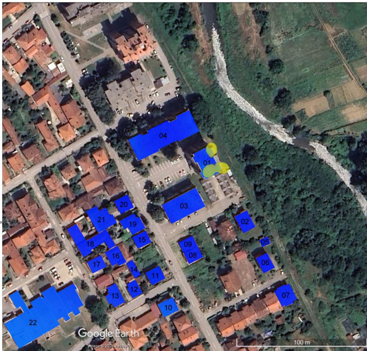
Слика 4.14. Фактор изложености унутар објеката када сви радио-системи оператора Cetin раде максималним капацитетом
