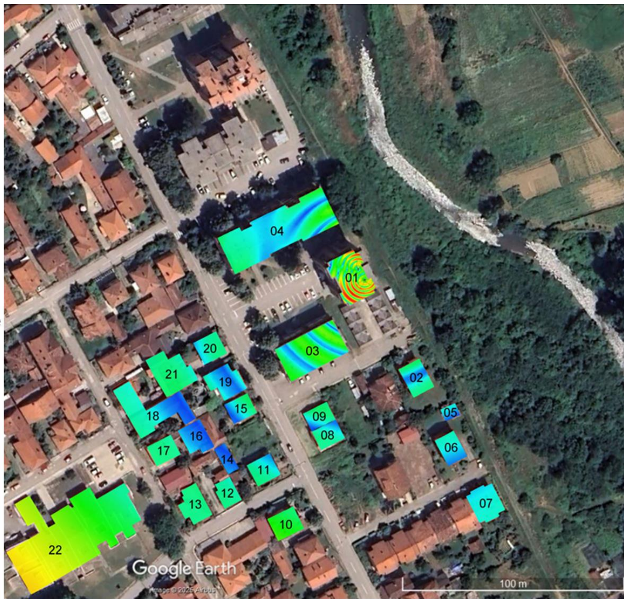
Слика 4.13. Јачина електричног поља унутар објеката када радио-систем LTE1800 оператора Cetin ради максималним капацитетом
