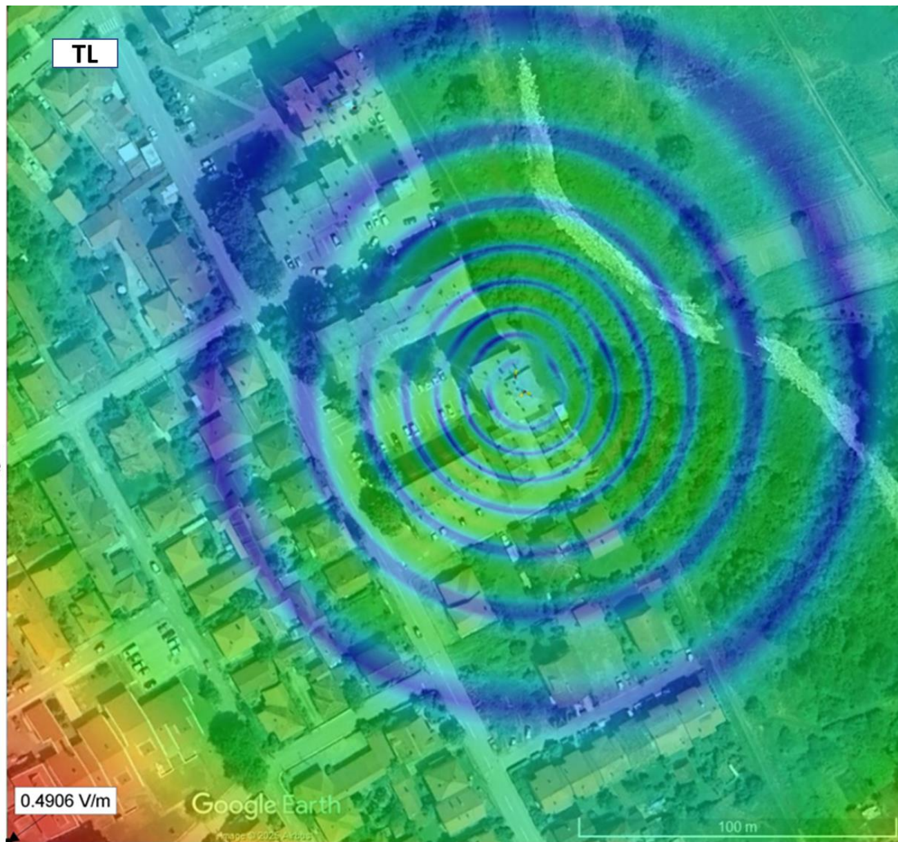
Слика 4.4. Јачина електричног поља на тлу, на јавном подручју, када радио-систем UMTS2100 оператора Cetin ради максималним капацитетом
