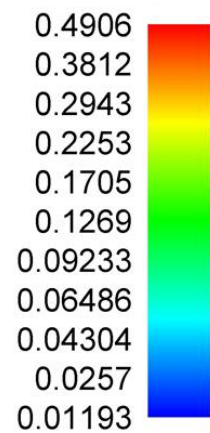
Слика 4.4. Јачина електричног поља на тлу, на јавном подручју, када радио-систем UMTS2100 оператора Cetin ради максималним капацитетом
