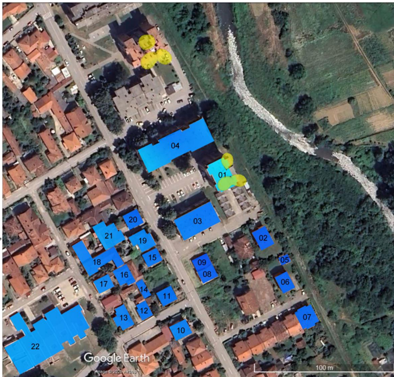
Слика 4.15. Фактор изложености унутар објекта када сви радио-системи свих оператора раде максималним капацитетом
