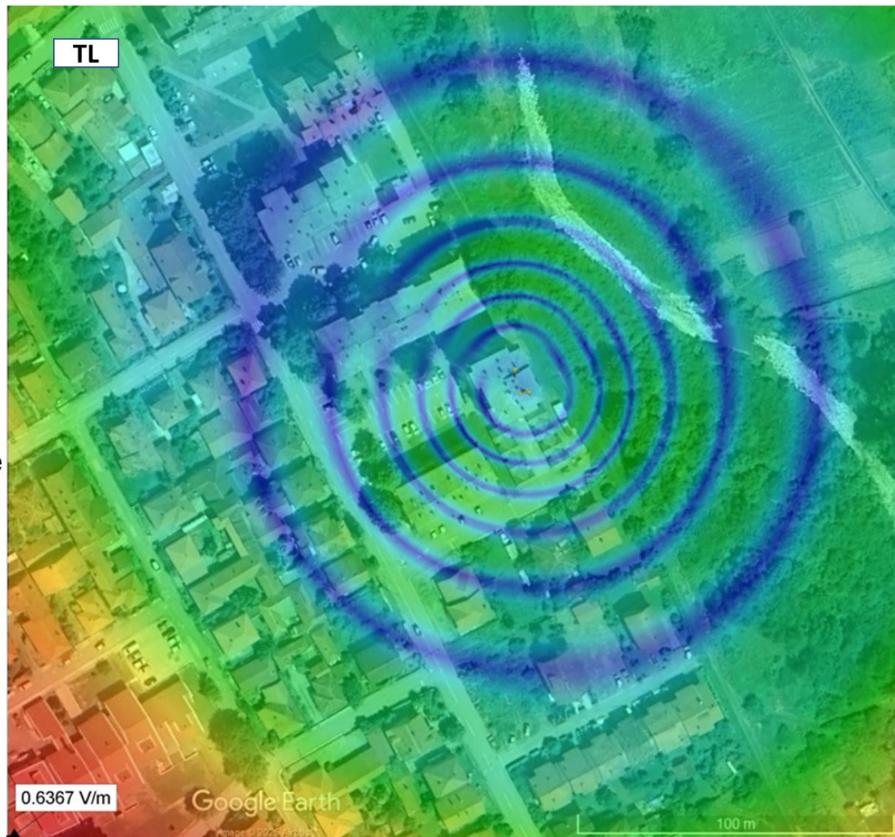
Слика 4.3. Јачина електричног поља на тлу, на јавном подручју, када радио-систем UMTS900 оператора Cetin ради максималним капацитетом
