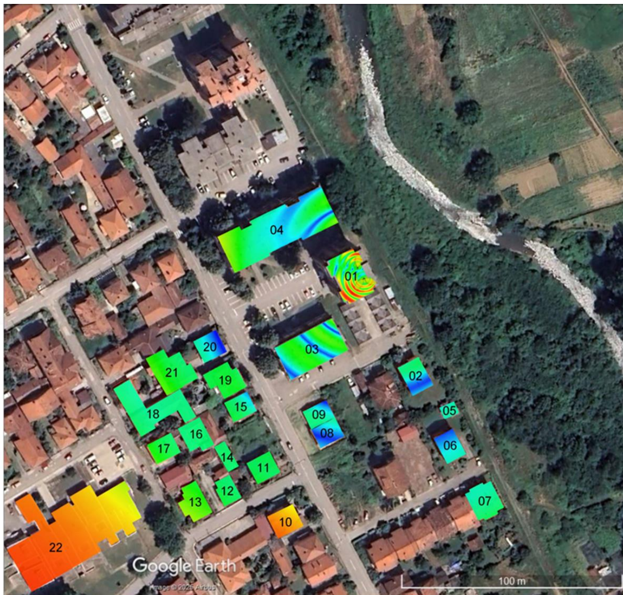
Слика 4.12. Јачина електричног поља унутар објекта када радио-систем LTE800 оператора Cetin ради максималним капацитетом
