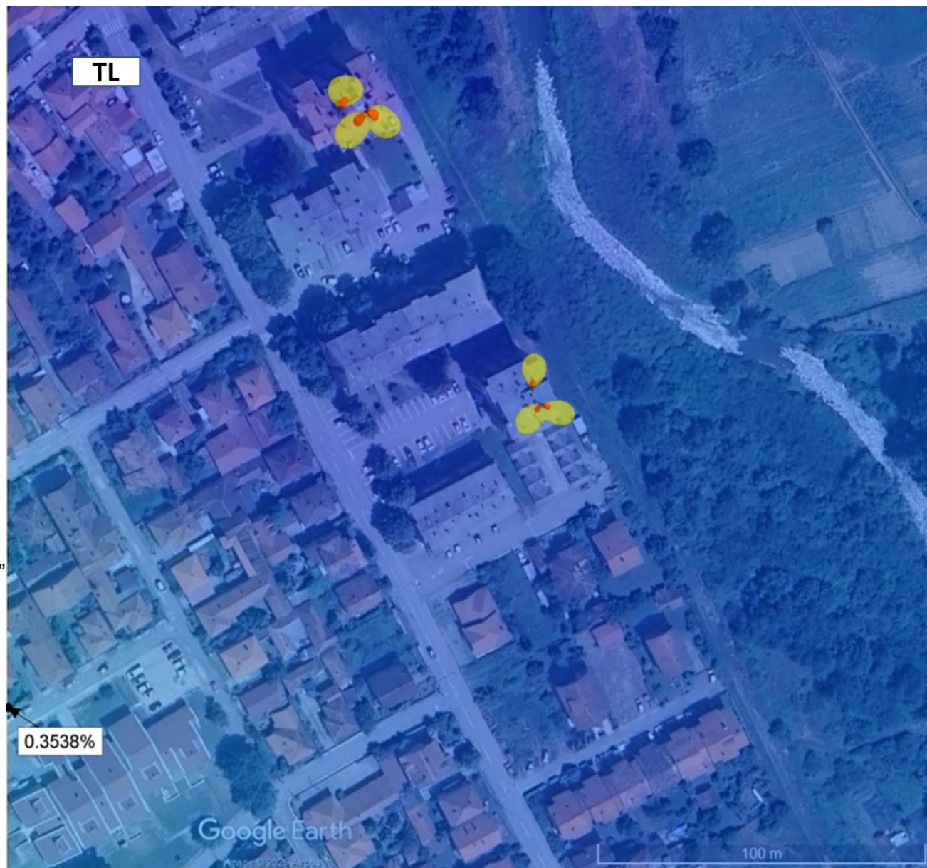
Слика 4.8. Фактор изложености на тлу, на јавном подручју, када сви радио-системи свих оператора раде максималним капацитетом
