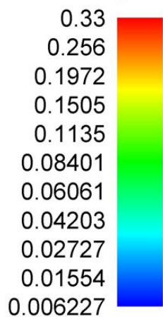
Слика 4.10. Јачина електричног поља унутар објекта када радио-систем UMTS900 оператора Cetin ради максималним капацитетом
