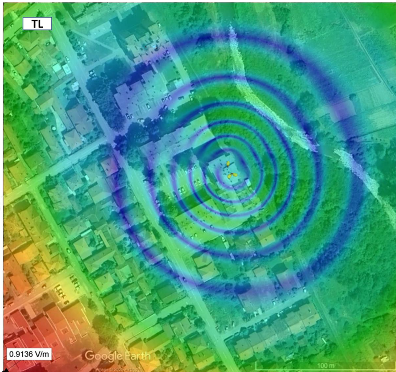
Слика 4.5. Јачина електричног поља на тлу, на јавном подручју, када радио-систем LTE800 оператора Setin ради максималним капацитетом
