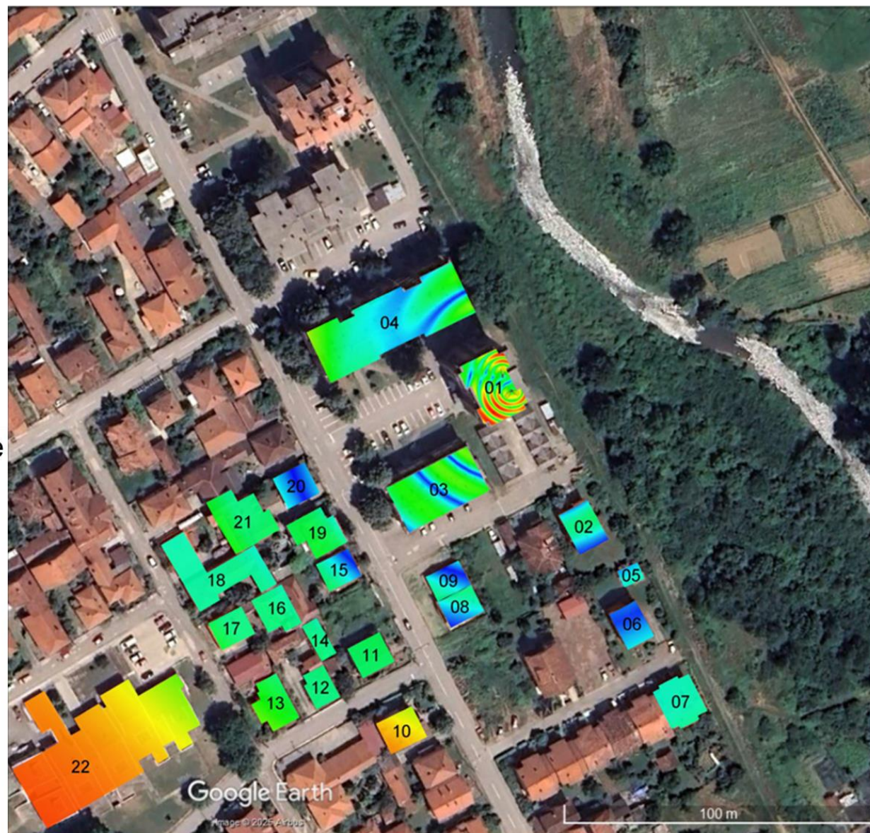
Слика 4.9. Јачина електричног поља унутар објекта када радио-систем GSM900 оператора Cetin ради максималним капацитетом
