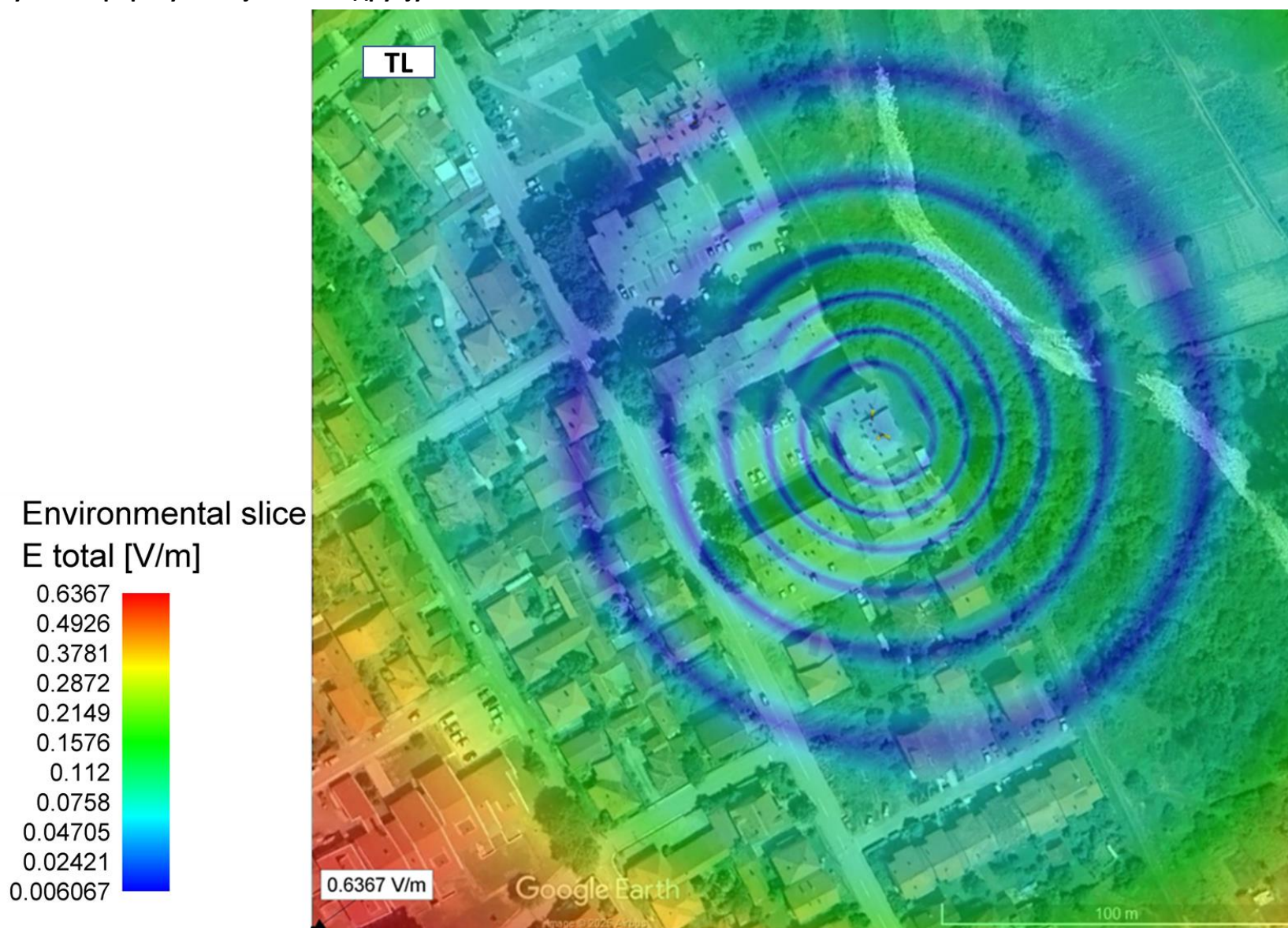
Слика 4.2. Јачина електричног поља на тлу, на јавном подручју, када радио-систем GSM900 оператора Setin ради максималним капацитетом
