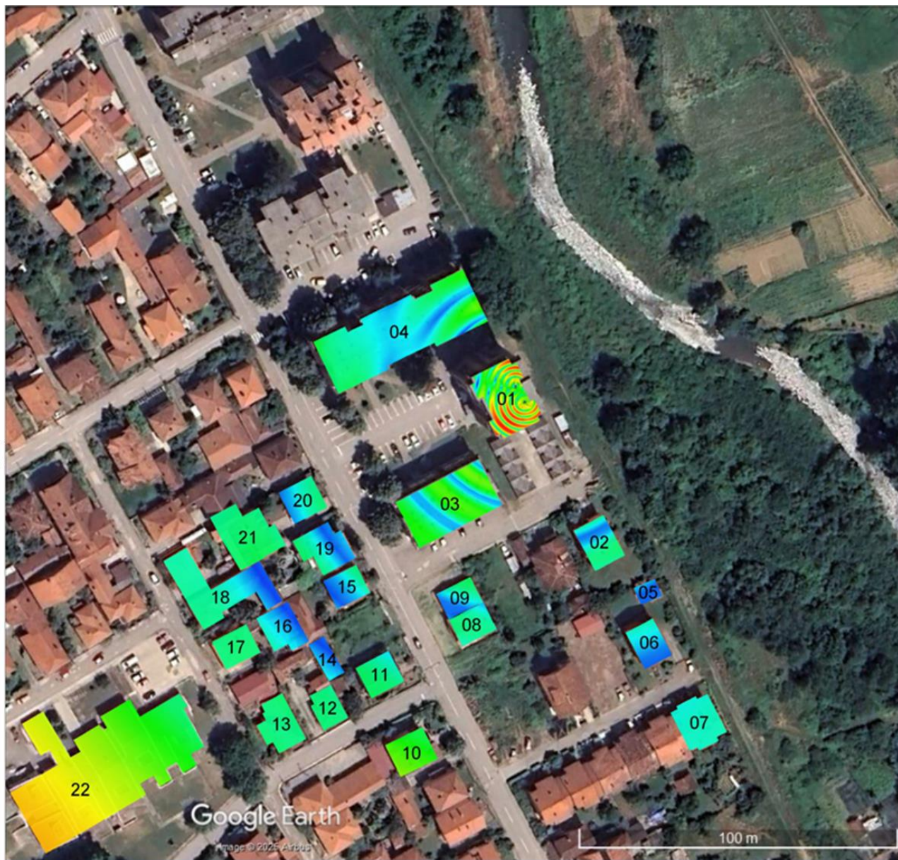
Слика 4.11. Јачина електричног поља унутар објекта када радио-систем UMTS2100 оператора Setin ради максималним капацитетом
